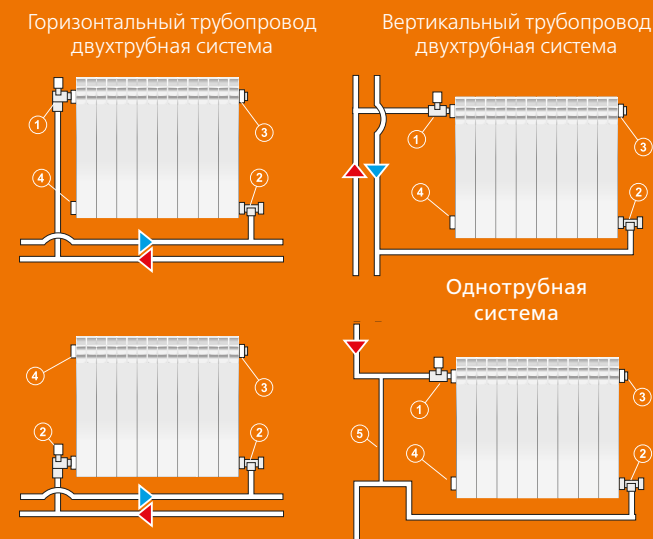
РИС. 2. РЕКОМЕНДУЕМЫЕ СХЕМЫ ПОДКЛЮЧЕНИЯ РАДИАТОРА К СИСТЕМЕ ОТОПЛЕНИЯ
