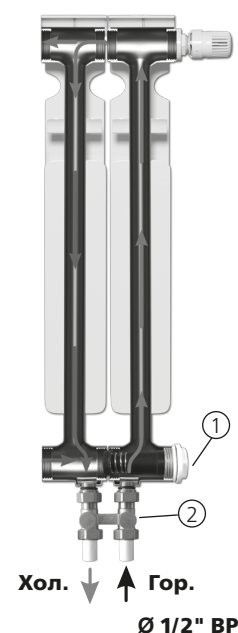
РИС. 3.3 ВИД РАДИАТОРА RADENA bimetall® VC500, VC350.
