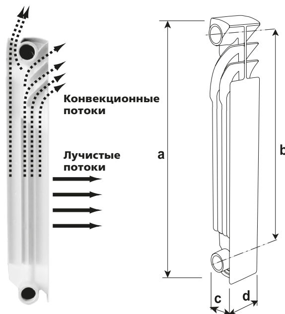
РИС. 3.4 ТЕПЛОВЫЕ ПОТОКИ И ГАБАРИТНЫЕ РАЗМЕРЫ РАДИАТОРА.
