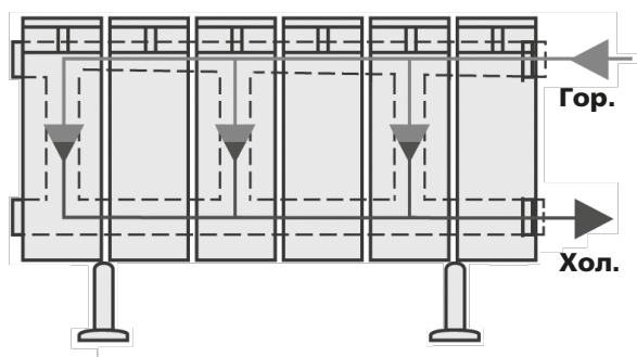
РИС. 3.2 ВИД РАДИАТОРА RADENA bimetall® CS150.
