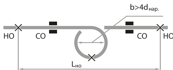
О-образный компенсатор
